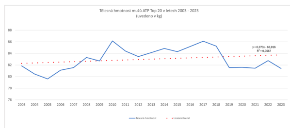
Graf 2 Vývoj a trend tělesné hmotnosti ATP mužů Top 20 v letech 2003–2023
