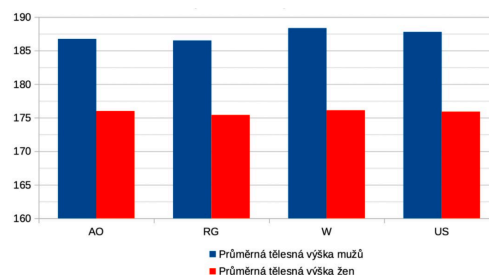
Graf 5 Tělesná výška čtvrtfinalistů mužů a žen na grandslamových turnajích v letech 2003–2023
