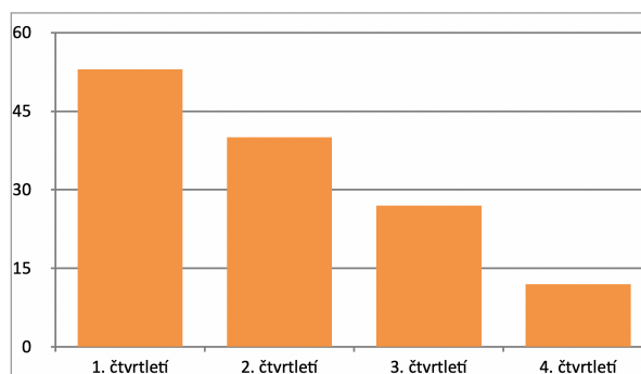
Graf 1 Rozložení četnosti dat narození hráčů (n = 132) v jednotlivých čtvrtletích (%) při World Junior Tennis Finals 2007–2009 v Prostějově (Zháněl et al., 2011)
